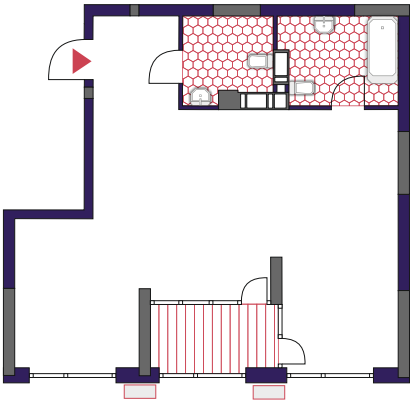
План квартири без перегородок
